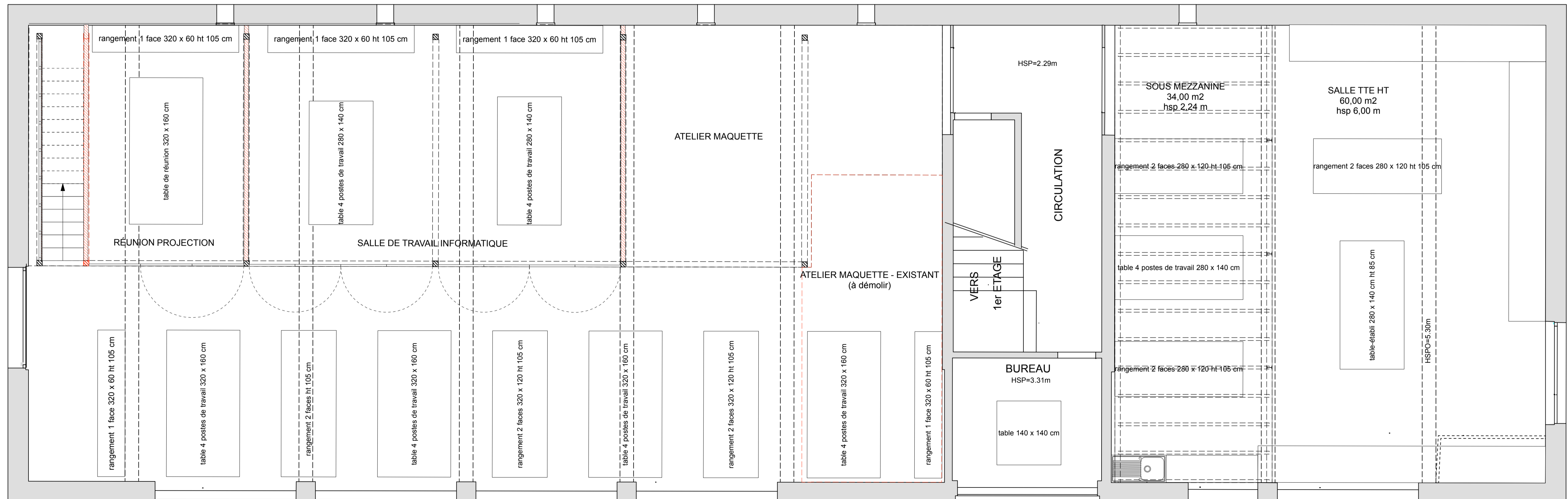
PLAN DU 1er ETAGE
